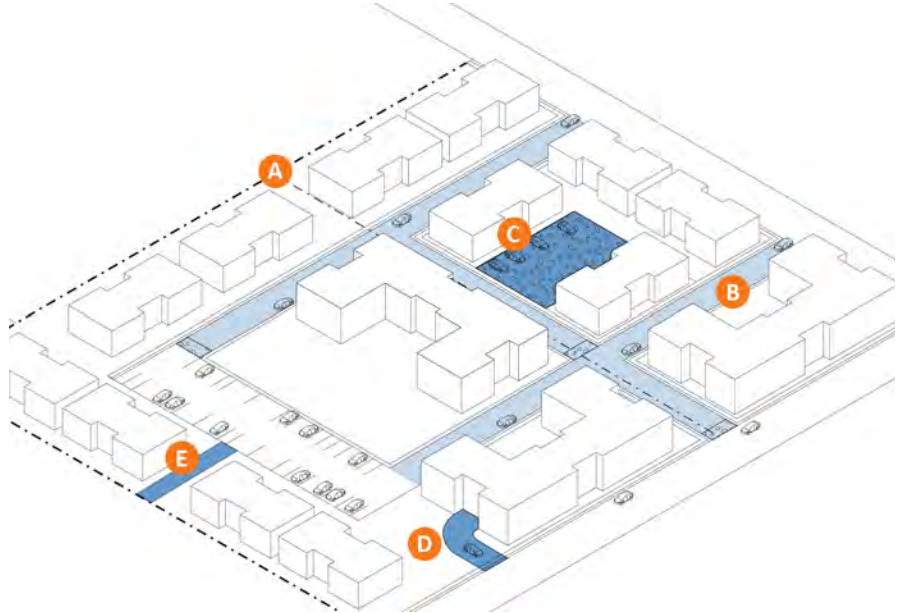
Figure 6.2: Parcel Subdivision
